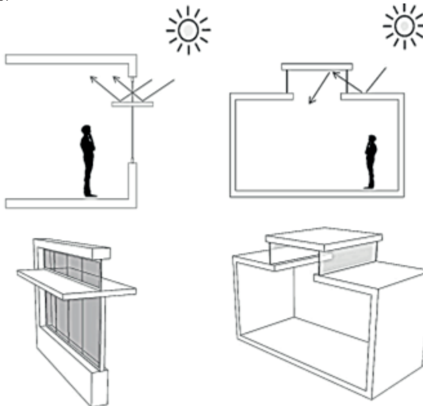
Figura 21. Representação de prateleira de luz: em corte (acima) e perspectiva (abaixo).
