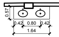
DETALHE VEST. FUNC. FEMININO ESCALA 1:100
