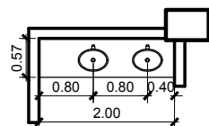
DETALHE SANITÁRIO FEM. - SALÃO VIP ESCALA 1:100
