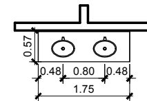
DETALHE VESTIÁRIO CASA PNE ESCALA 1:100
