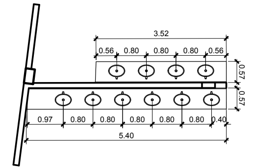
DETALHE SANITÁRIO MASCULINO 1 ESCALA 1:100
