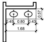
DETALHE SANITÁRIO FEMININO - IMPRENSA ESCALA 1:100
