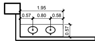
DETALHE SANITÁRIO MASC. - SALÃO VIP ESCALA 1:100
