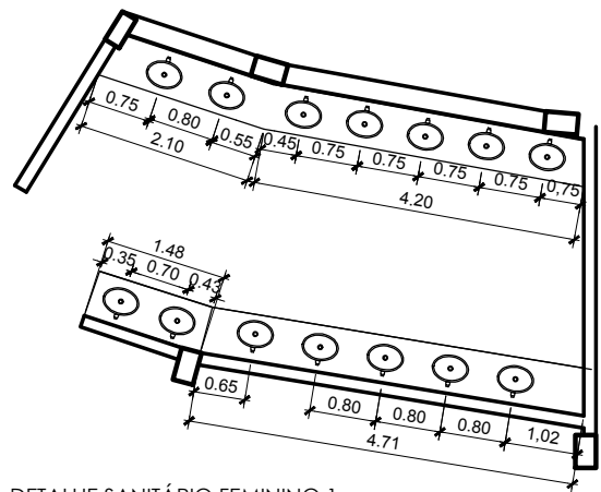
DETALHE SANITÁRIO FEMININO 1 ESCALA 1:100
