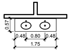
DETALHE VEST. VISITANTES PNE ESCALA 1:100
