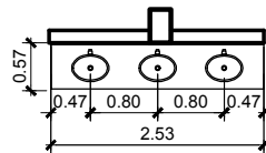
DETALHE VESTIÁRIO CASA ESCALA 1:100
