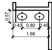
DETALHE SANITÁRIO MASCULINO - IMPRENSA ESCALA 1:100
