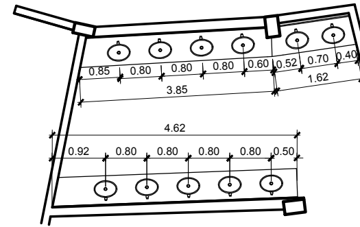
DETALHE SANITÁRIO FEMININO 2 ESCALA 1:100
